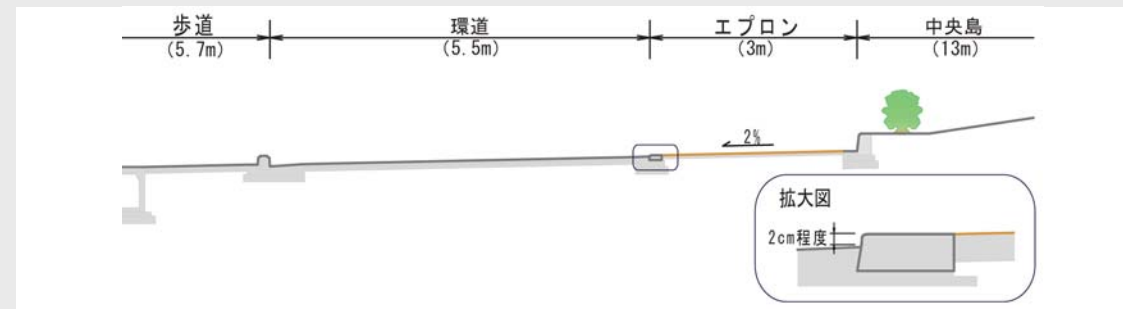
↑ カラー舗装と段差を設けることで、視覚的・物理的に還道部の直線的な通過の抑制を促す。大型車が乗り入れ可能な高さとするこで、大型車の内輪差を補う。
