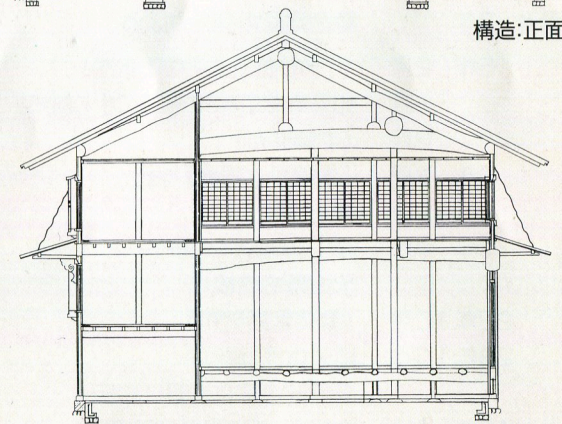
構造：側面図
