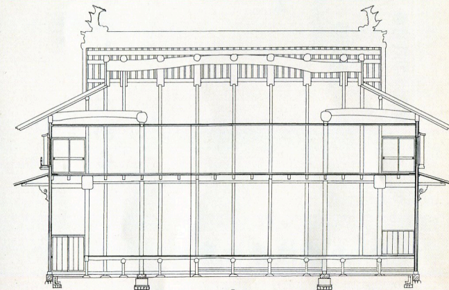
構造：正面図
